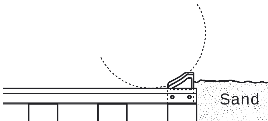
Figur 0-1. Stopklodser.
